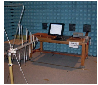
EMI/EMV
